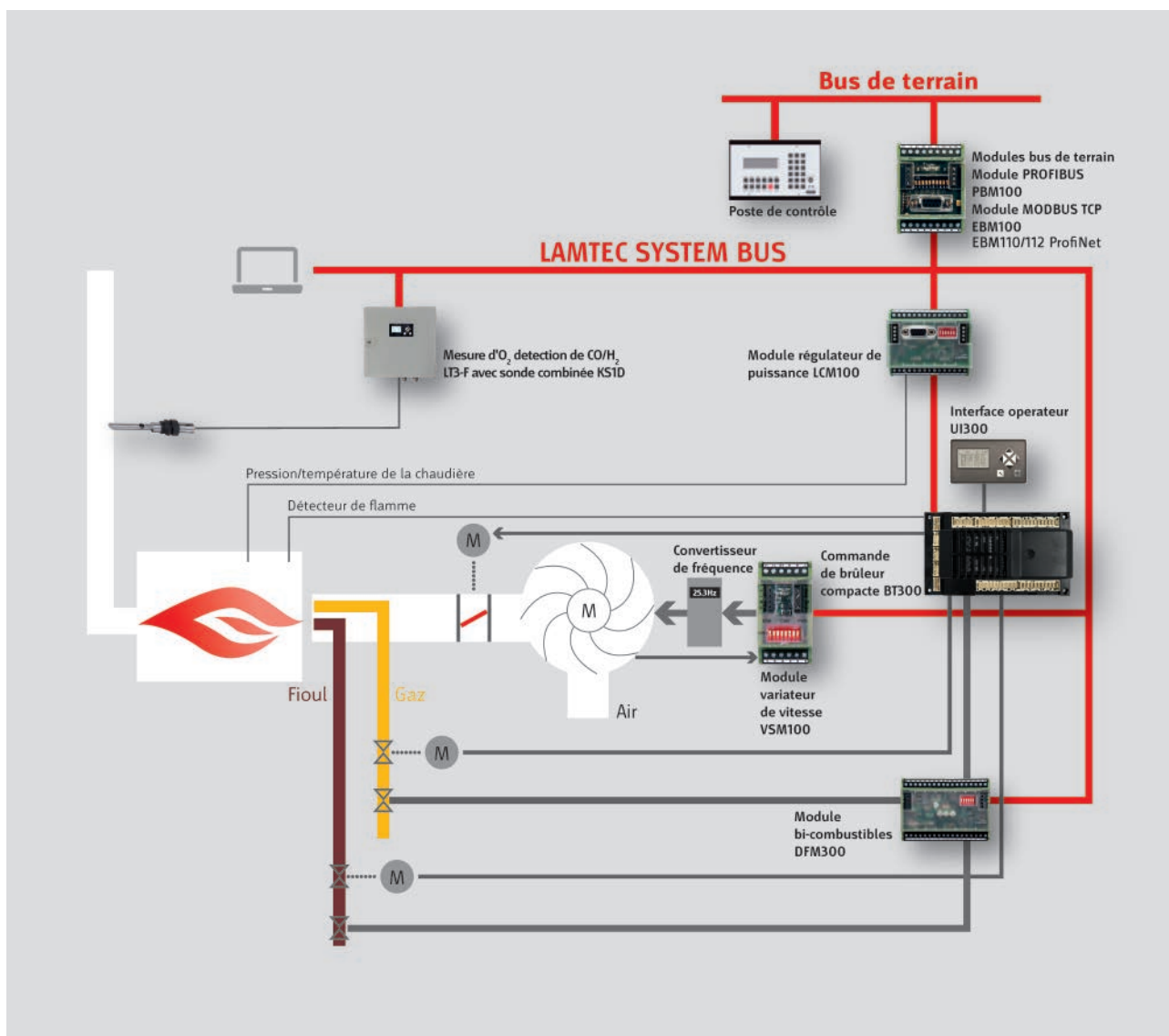
Aperçu des fonctions BT340/341.
