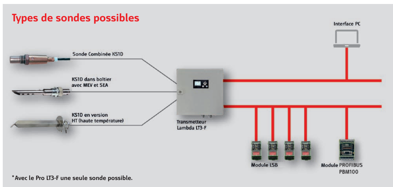
Aperçu de fonctionnement LT3-F avec KS1D-Ex.
