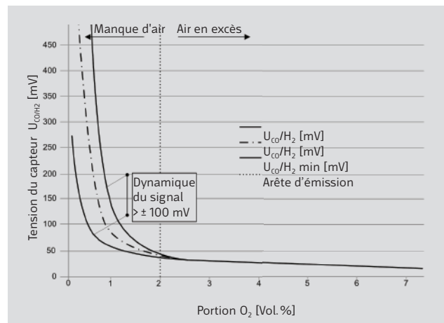
Dynamique du signal d'électrode CO_e U_{CO/H_2} dans la zone de manque d'air.
