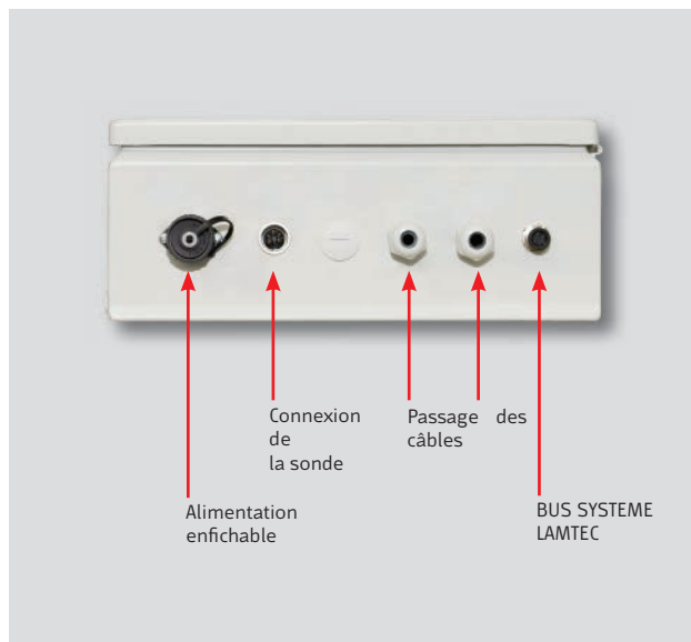
Connecteurs LT3-F sur le dessous.
