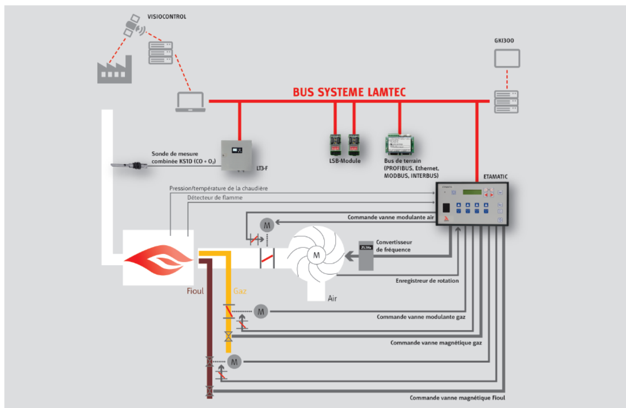
Vue d'ensemble des fonctions ETAMATIC / ETAMATIC S.
