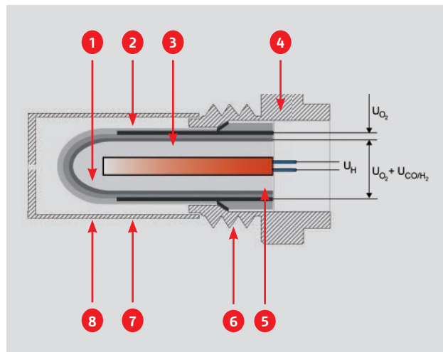
Structure de principe de la Sonde Combinée LAMTEC KS1D
