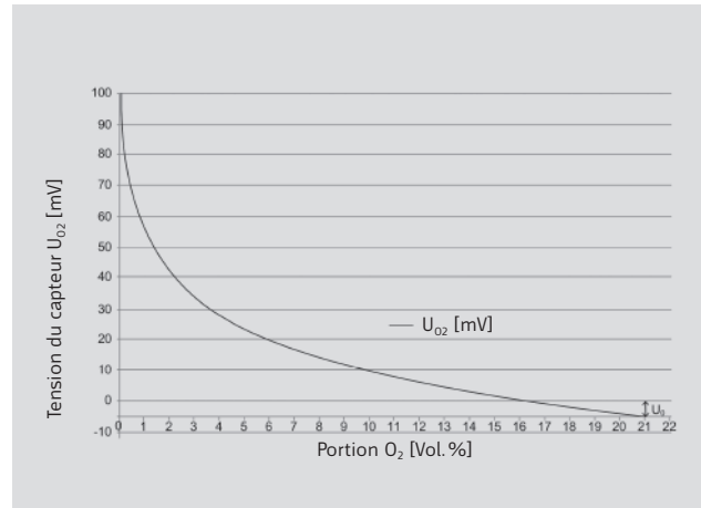
Caractéristique de Nernst du capteur U_s = f(O_2)
