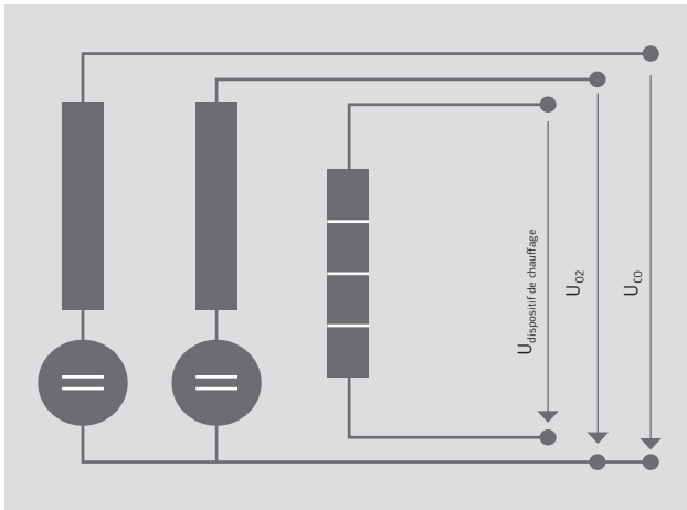
Schéma de connexion de rechange simple KS1D.
