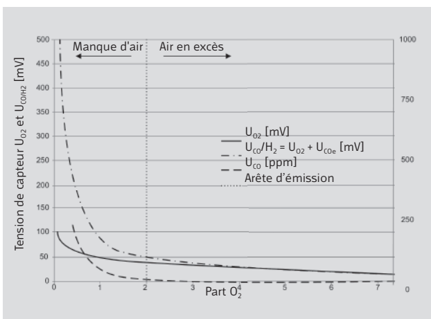
Tracé typique des deux tensions de capteur KS1D
